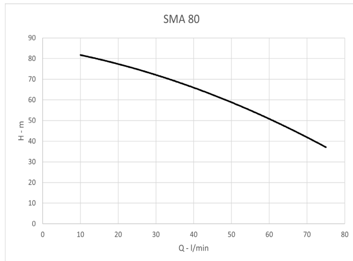
Leistungskurve SMA80
